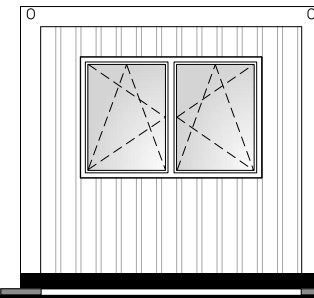
Achtergevel
