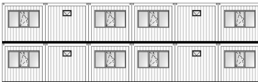
Achtergevel
