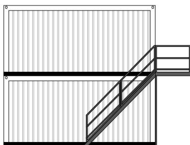
Linkergevel
